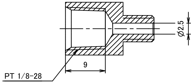
A-A (2:1)
